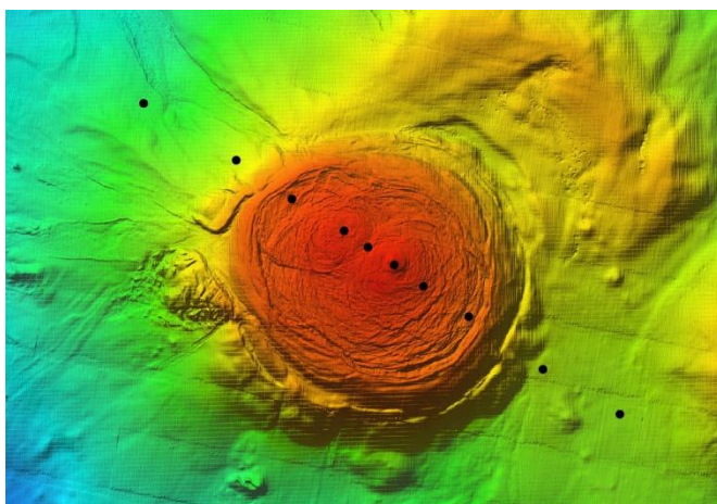
Abbildung 3: AUV-Karte des Sartori Schlammvulkans. Die 10 schwarzen Punkte in der Karte markieren die 10 Lokationen, an denen jeweils ein 5 m tiefes Wärmestromprofil gemessen wurde.
