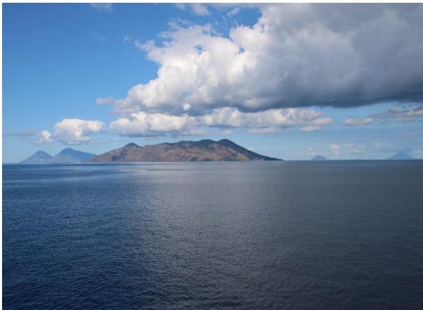
Abbildung 1: Blick von FS SONNE auf die Liparischen Inseln im Tyrrhenischen Meer mit Lipari im Vordergrund, Paneria und Stromboli rechts daneben (© Julia Kraft).
