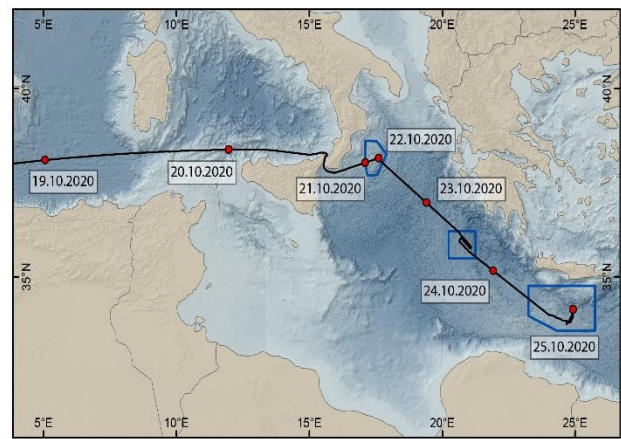
Abbildung 2: Fahrtroute der vergangenen Woche vom westlichen in das östliche Mittelmeer mit Lage der 3 Arbeitsgebiete.
