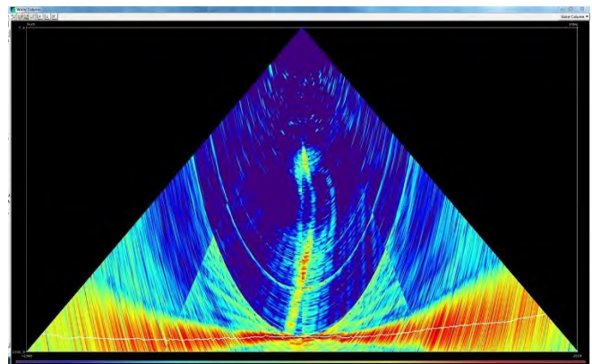
Abbildung 4: Wie auch in früheren Untersuchungen gezeigt, ist der Haakon Mosby Schlammvulkan ein recht aktiver Vulkan. Er ist für Gasemissionen bekannt, die wir im Multibeam-Fächer deutlich durch mehrere gebogene „Flares“ im Zentrum erkennen konnten.
