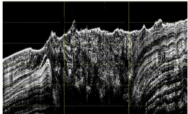
Parasound-Profil durch den Schlammvulkan vor der Sambesi-Mündung (© MARUM – Zentrum für Marine Umweltwissenschaften, Universität Bremen)
