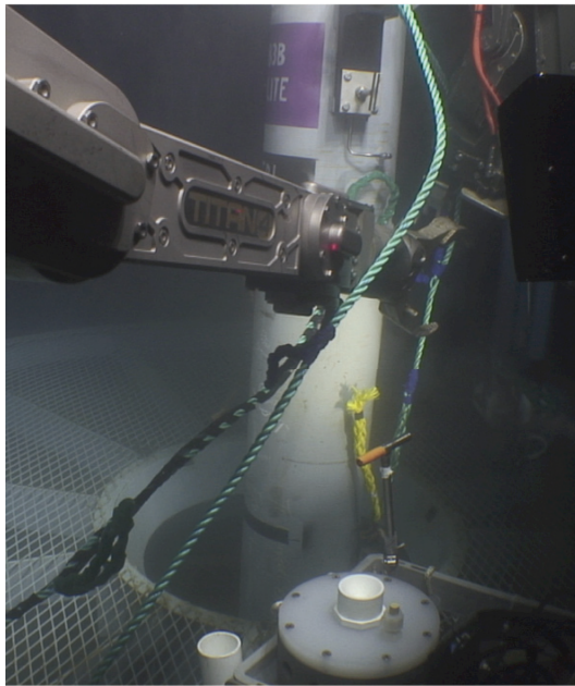
Bild 3: In Bohrung U1383B wurde ein CORK Observatorium von Jason installiert und mit einem OSMO-Set bestückt, das in 50 m Tiefe Proben nimmt (Quelle: WHOI)
