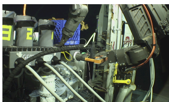
Bild 1: Jason schließt den GeoMICROBE-Schlitten ans Observatorium in Bohrloch 1383C an (Quelle: WHOI).
