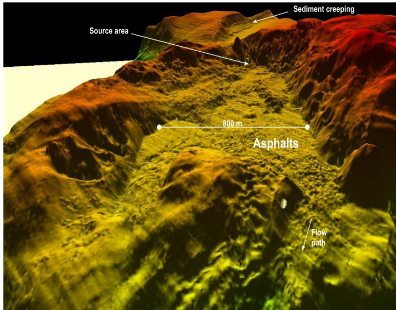
Abb. 1: Perspektivische Darstellung des Reliefs eines Asphaltvulkans anhand von Fächerlotdaten des AUV. Der zentrale, etwa 800 m messende Bereich des Kraters scheint mit Asphalt bedeckt zu sein. Schweres Öl tritt vermutlich an der höchstgelegenen Stelle aus, füllt den Krater und fließt weiter dem Gefälle folgend.
