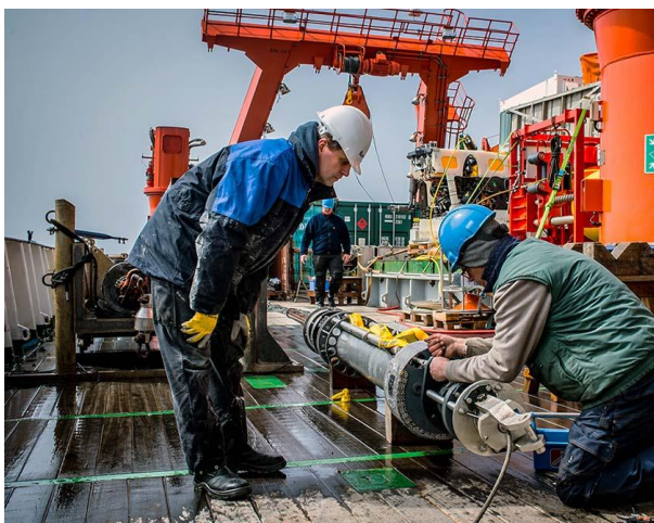
Abbildung 1: Das Autoklav-Kolbenlot DAPC wird nach Einsatz im Church Trog an Deck der METEOR auf seine Dichtigkeit hin untersucht.
